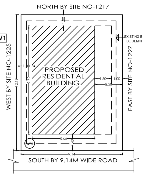
SITE PLAN 1:100
